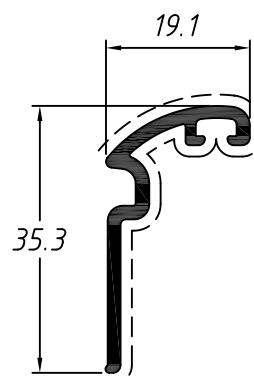
Tapa junta IN203 0,278 Kg/m
