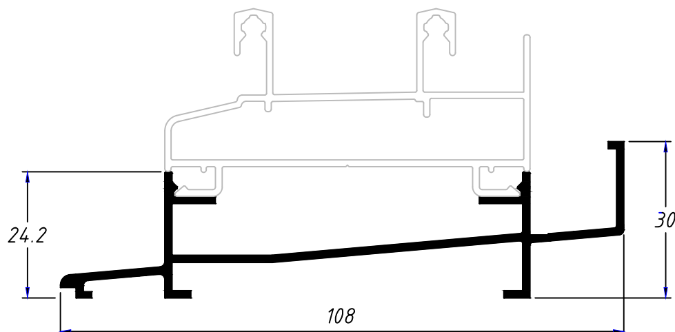
Marco para drenaje AK215 0,779 Kg/m
