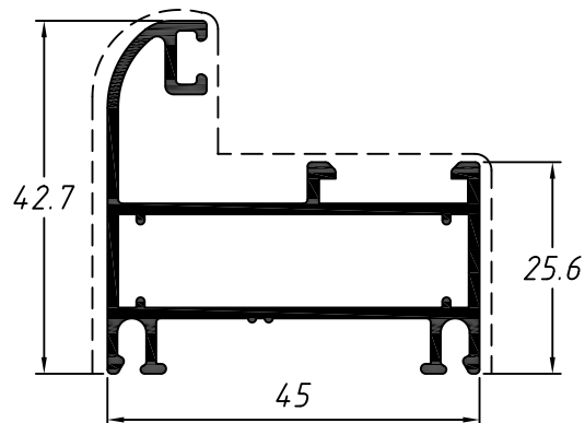
Marco liso perimetral proyectante
