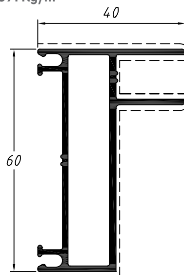
Parante lateral de 2 rieles
