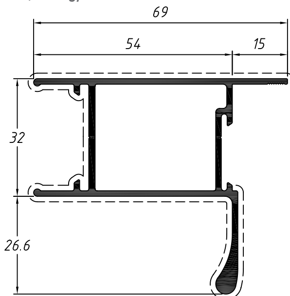
Hoja lateral y central con refuerzo
