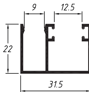
Guía inferior chica para 8mm CK321 0,308 Kg/m
