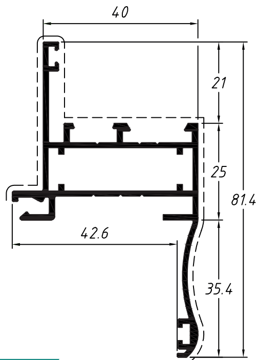
Marco perimetral combinable con corrediza
