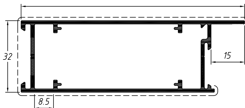
Hoja lateral y central reforzada batiente
