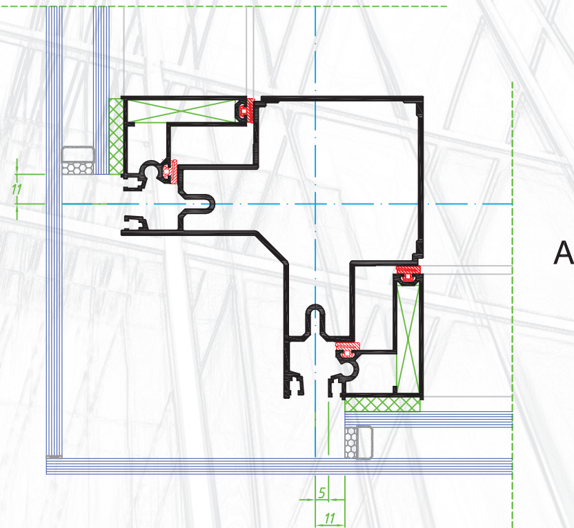
CORTE HORIZONTAL
