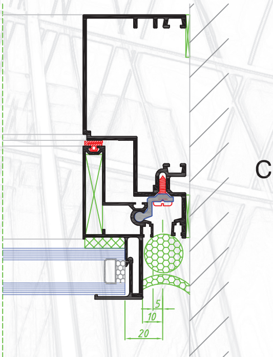
CORTE HORIZONTAL
