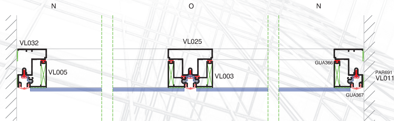
CORTE HORIZONTAL
