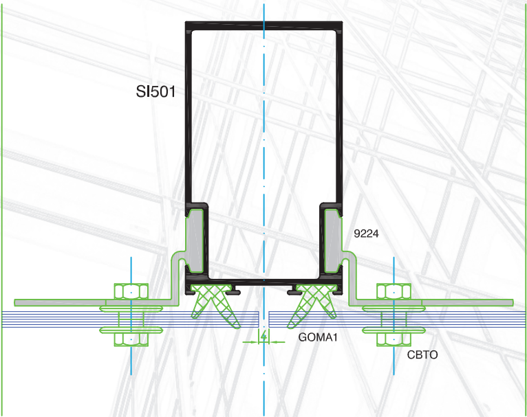
Detalle central de COLUMNA VIDRIO SIMPLE
