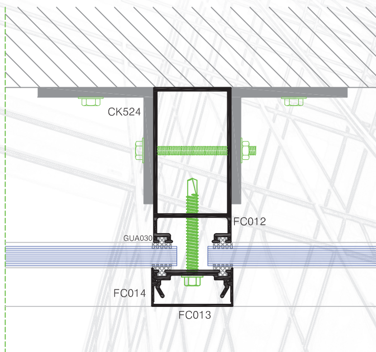
Detalle CENTRAL columna 80x40mm FC012 VIDRIO SIMPLE
