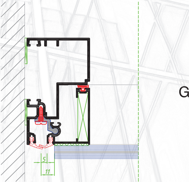
CORTE HORIZONTAL
