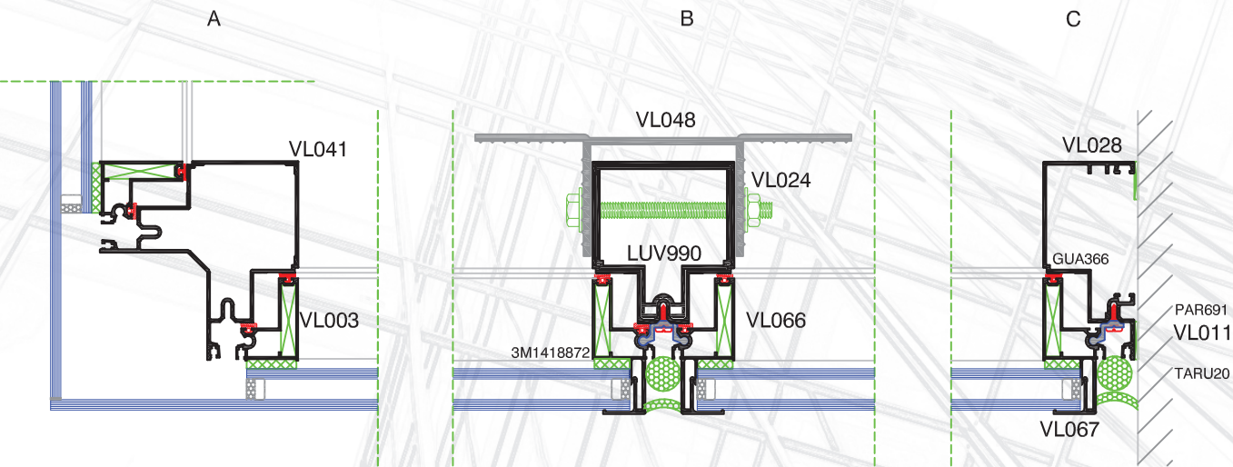
CORTE HORIZONTAL
