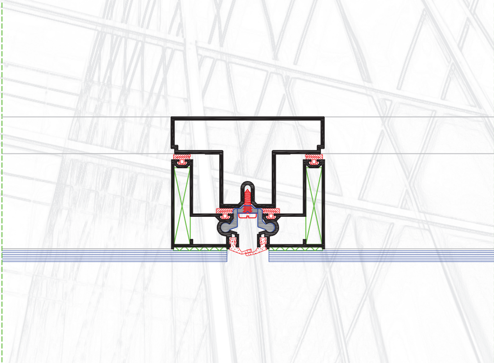
CORTE HORIZONTAL
