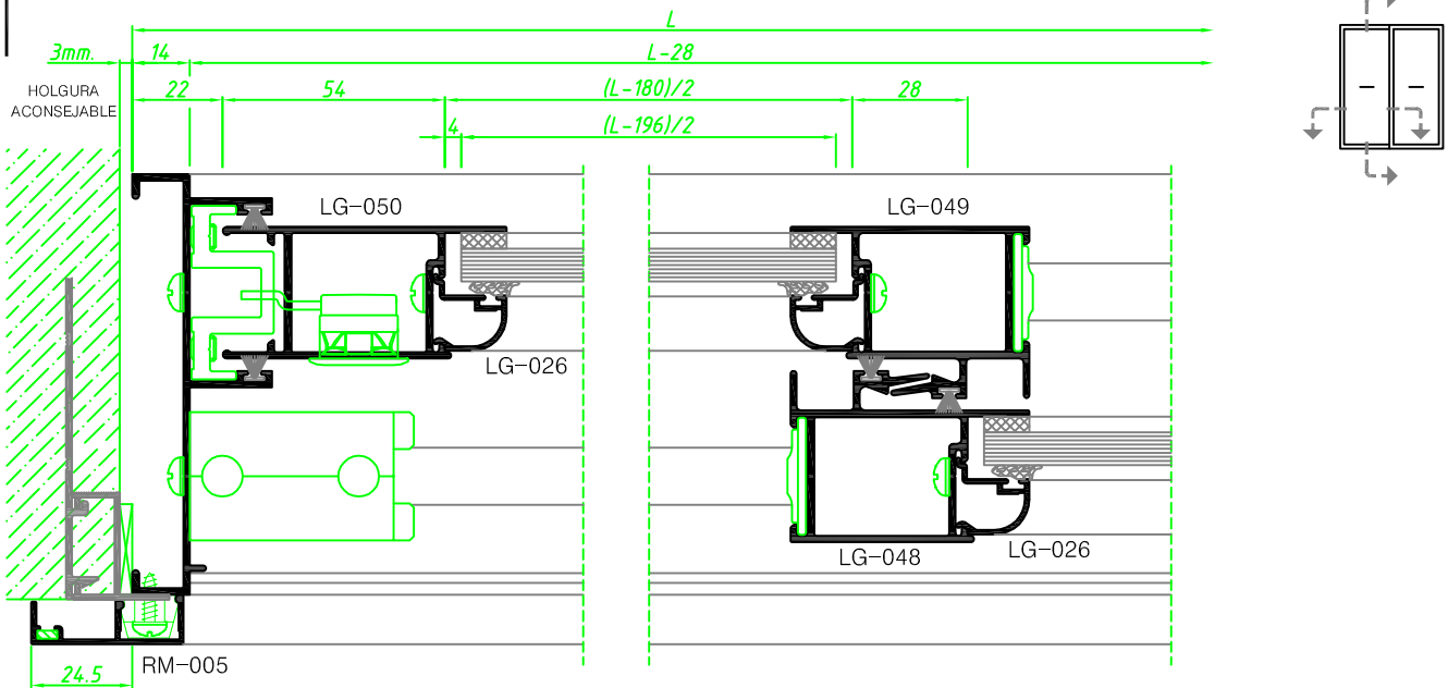
CORTE HORIZONTAL
