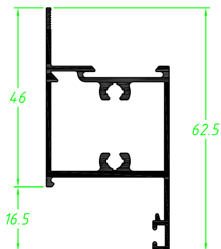
Marco para fijos a corte 45°
