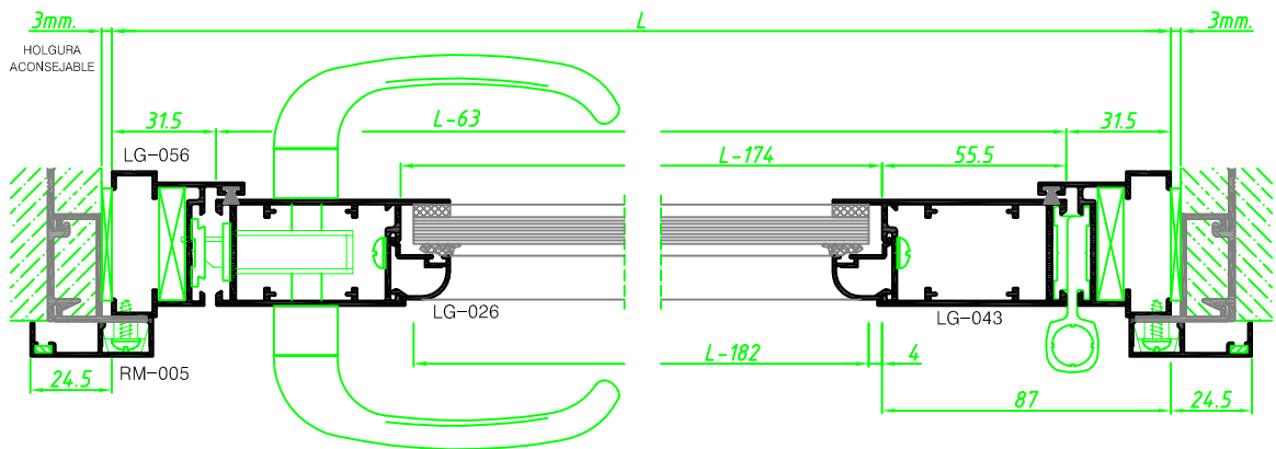
CORTE HORIZONTAL
