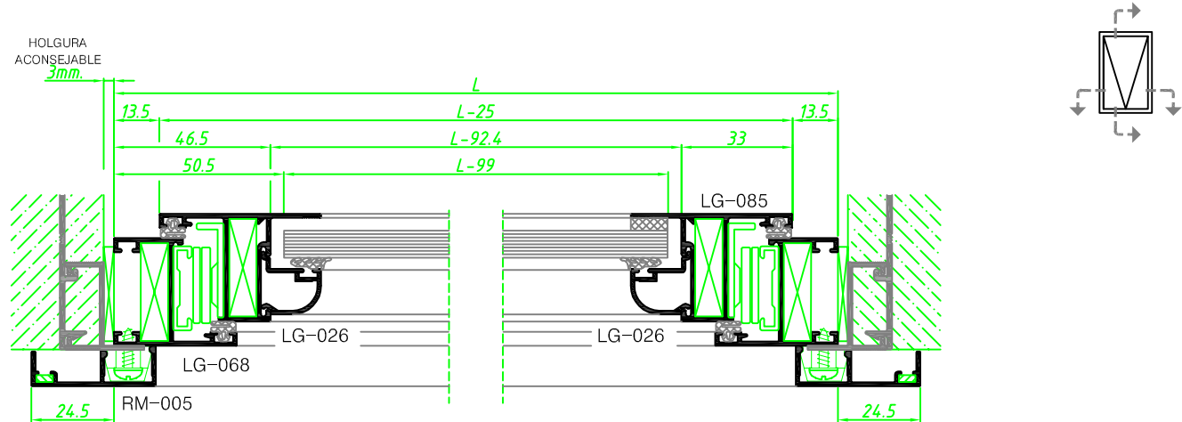
Encuentro lateral VENTANA PROYECTANTE CORTE a 45°
