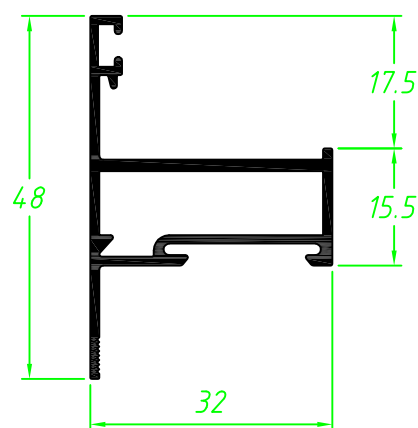
Columna divisoria atornillada para fijos
