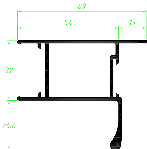
Hoja de enganche interno con tubular
