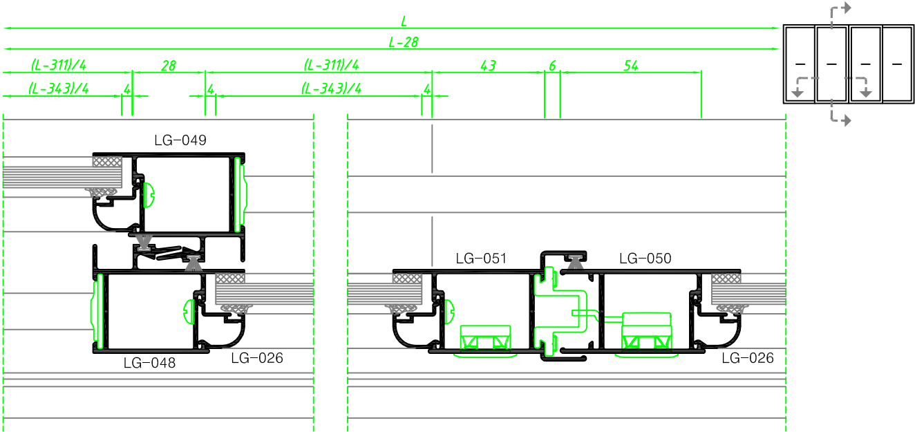
CORTE HORIZONTAL
