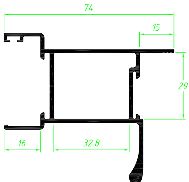
Hoja de enganche externo con tubular
