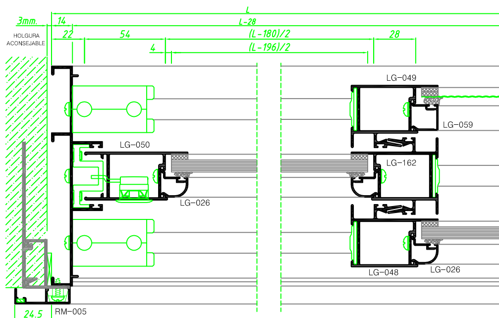
CORTE HORIZONTAL
