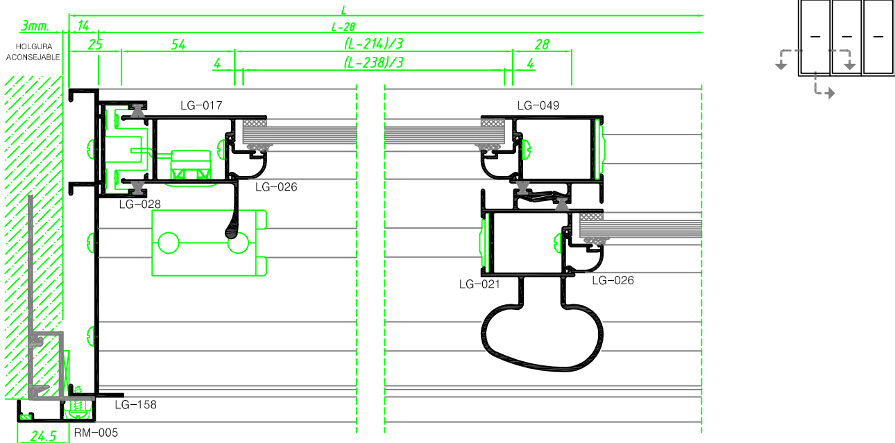
CORTE HORIZONTAL
