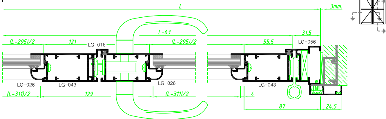
CORTE HORIZONTAL
