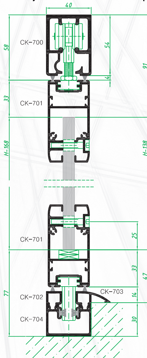
CORTE VERTICAL - VISTA ENGUIADOR PIVOTANTE
