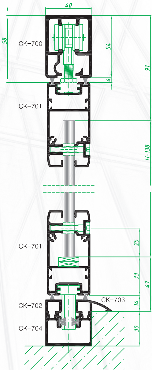
Encuentro INFERIOR y SUPERIOR Puerta Semi-Emprotada
