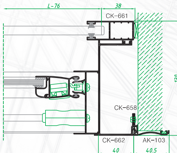
Encuentro Lateral con guía de 130 mm para persiana Manual
