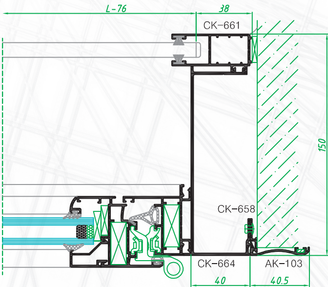
Encuentro Lateral con guía de 150mm para persiana Manual
