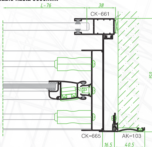
Encuentro Lateral con guía de 150mm para persiana a Motor
