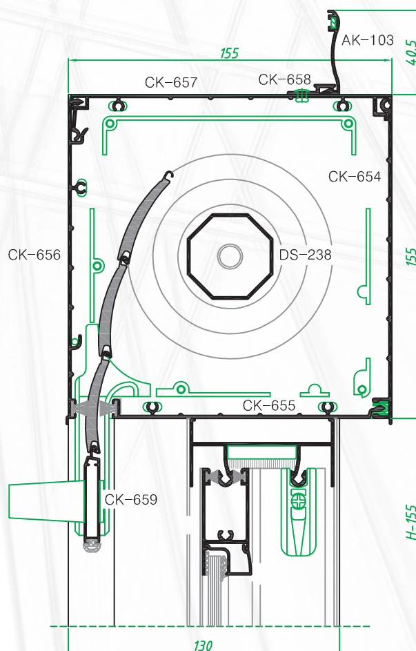
Encuentro vertical superior con eje de 41mm y caja de 155mm
