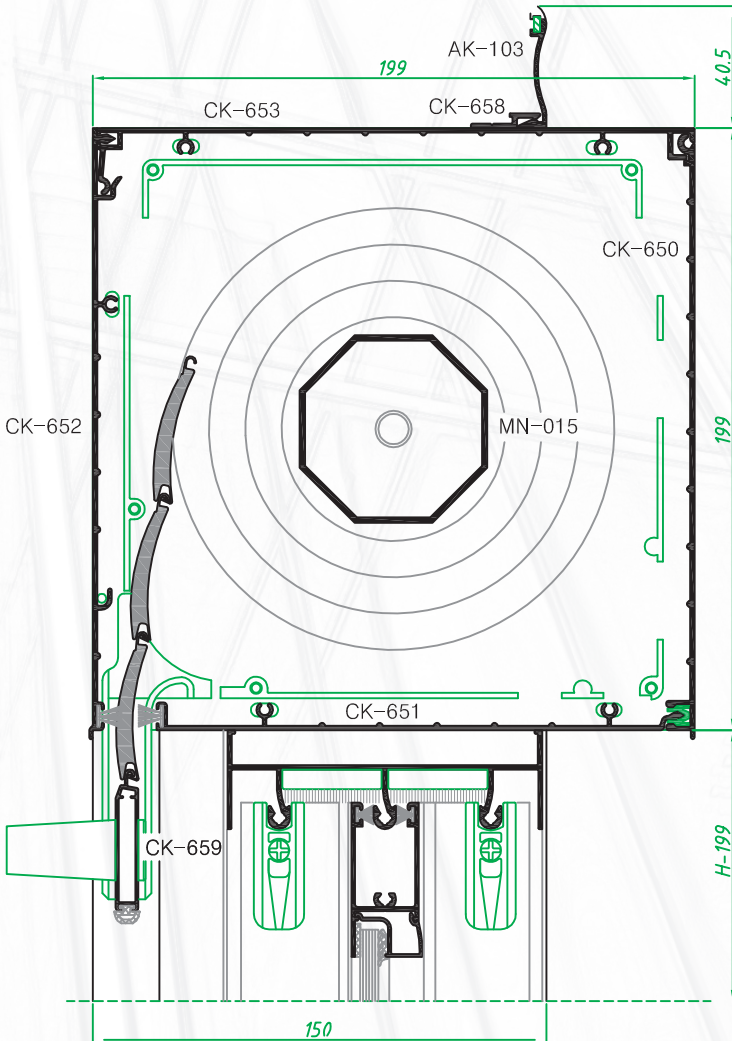
Encuentro vertical superior con eje de 62mm y caja de 200mm
