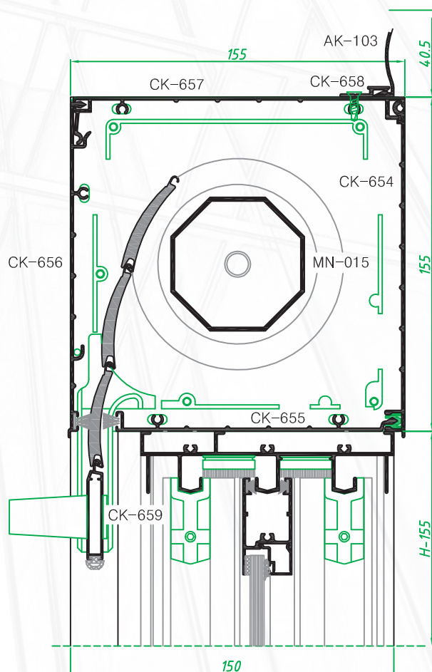
Encuentro vertical superior con eje de 62mm y caja de 155mm
