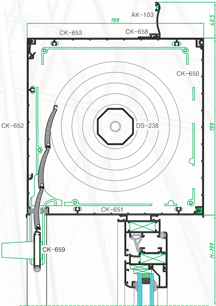
Encuentro vertical superior con eje de 41mm y caja de 200mm
