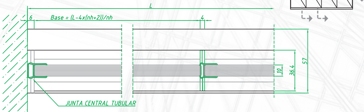
Encuentro INFERIOR y SUPERIOR Puerta Semi-Empotrada
