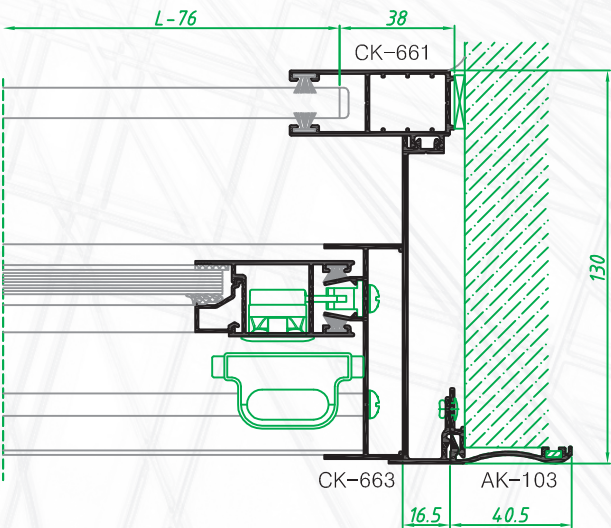
Encuentro lateral con guía de 130mm para persiana a motor
