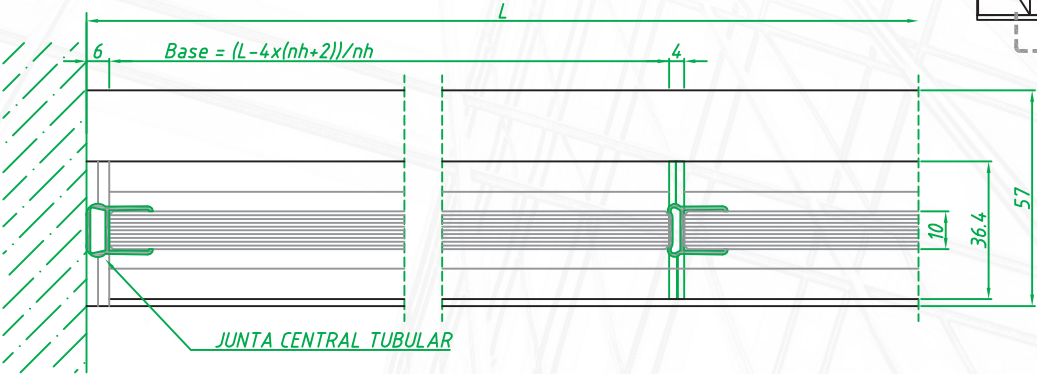
Encuentro INFERIOR y SUPERIOR Puerta Empotrada
