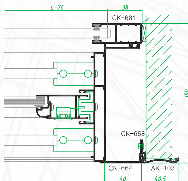
Encuentro Lateral con guía de 150mm para persiana Manual
