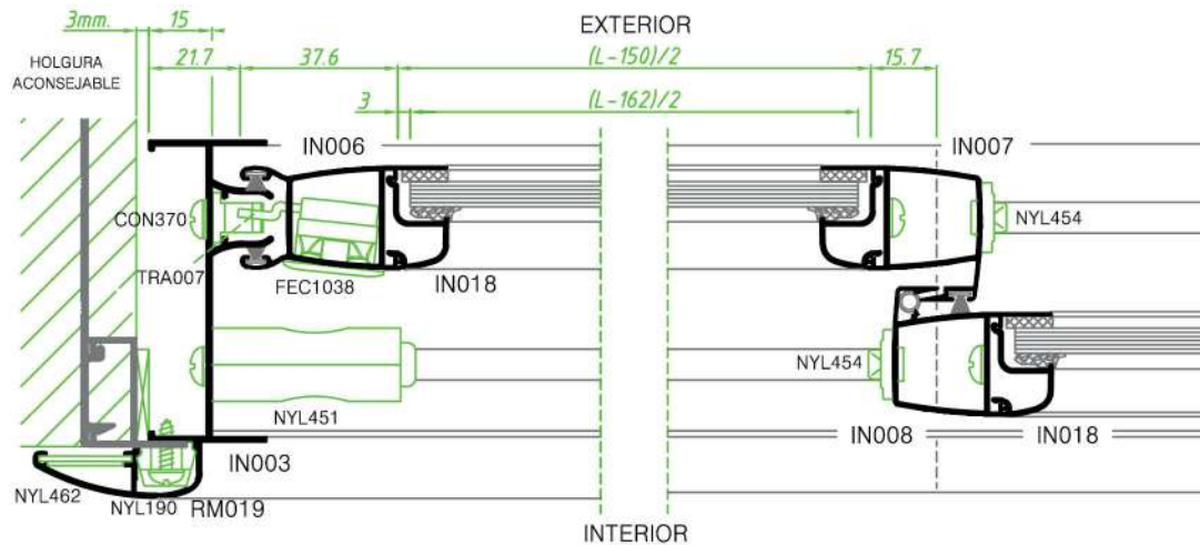
CORTE HORIZONTAL | ESC. 1:2
