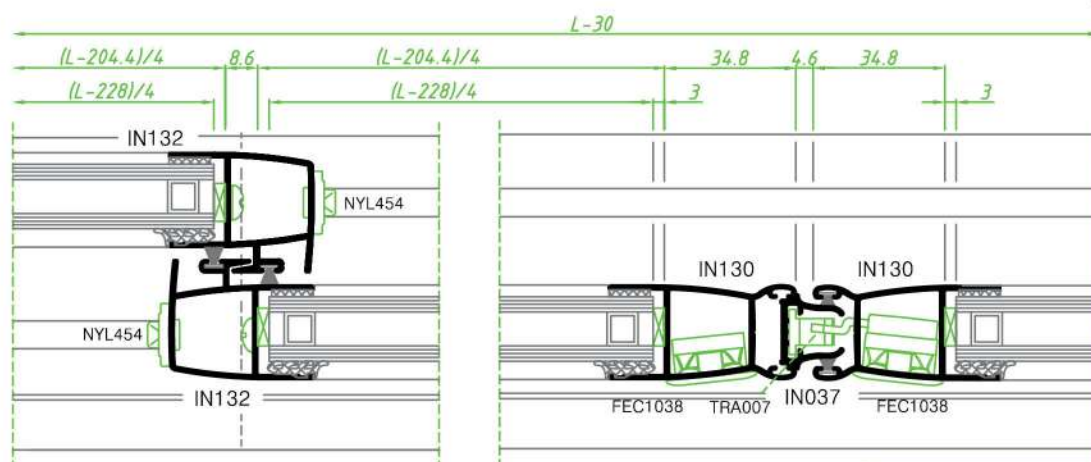
CORTE HORIZONTAL | ESC. 1:2
