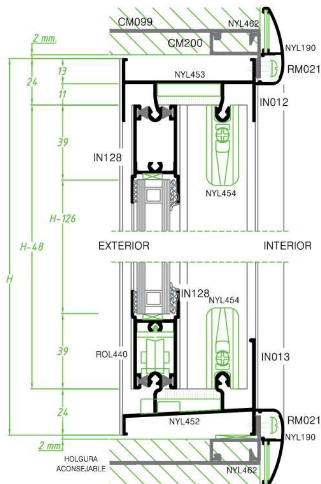
CORTE VERTICAL | ESC. 1:2
