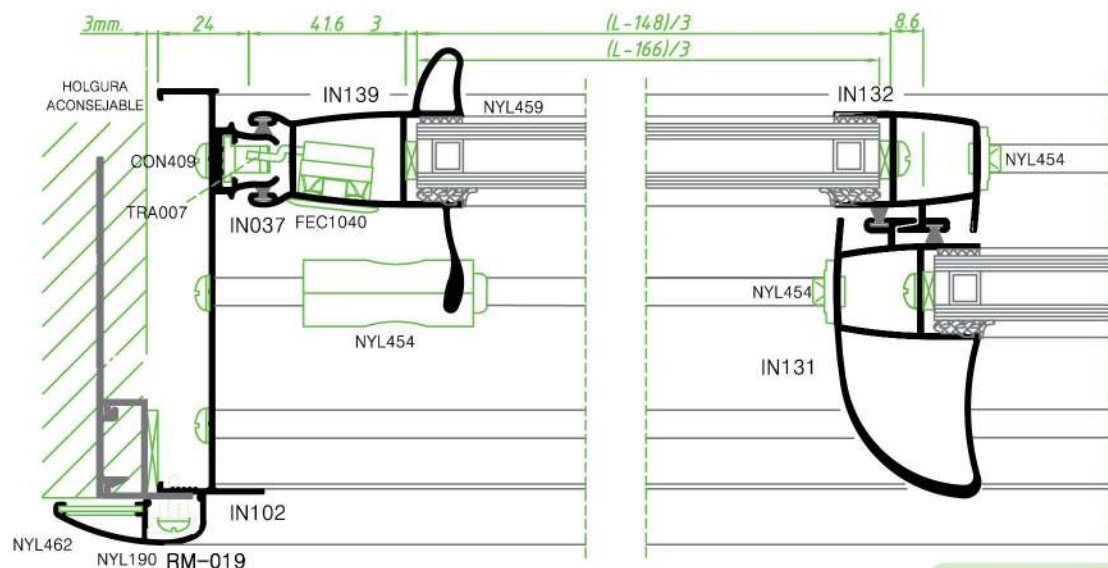
CORTE HORIZONTAL | ESC. 1:2
