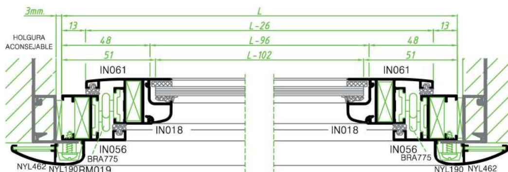
CORTE HORIZONTAL | ESC. 1:2
