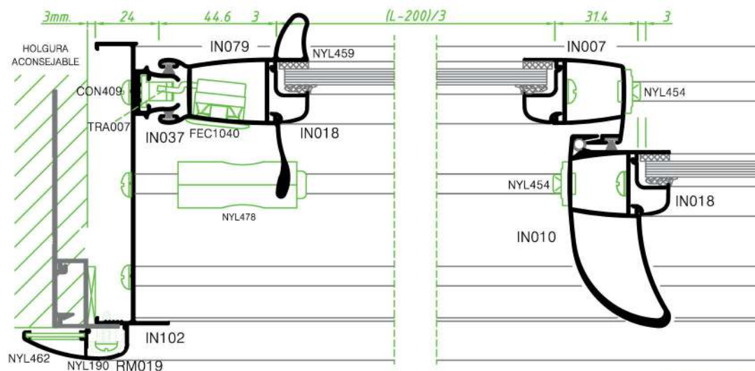
CORTE HORIZONTAL | ESC. 1:2
