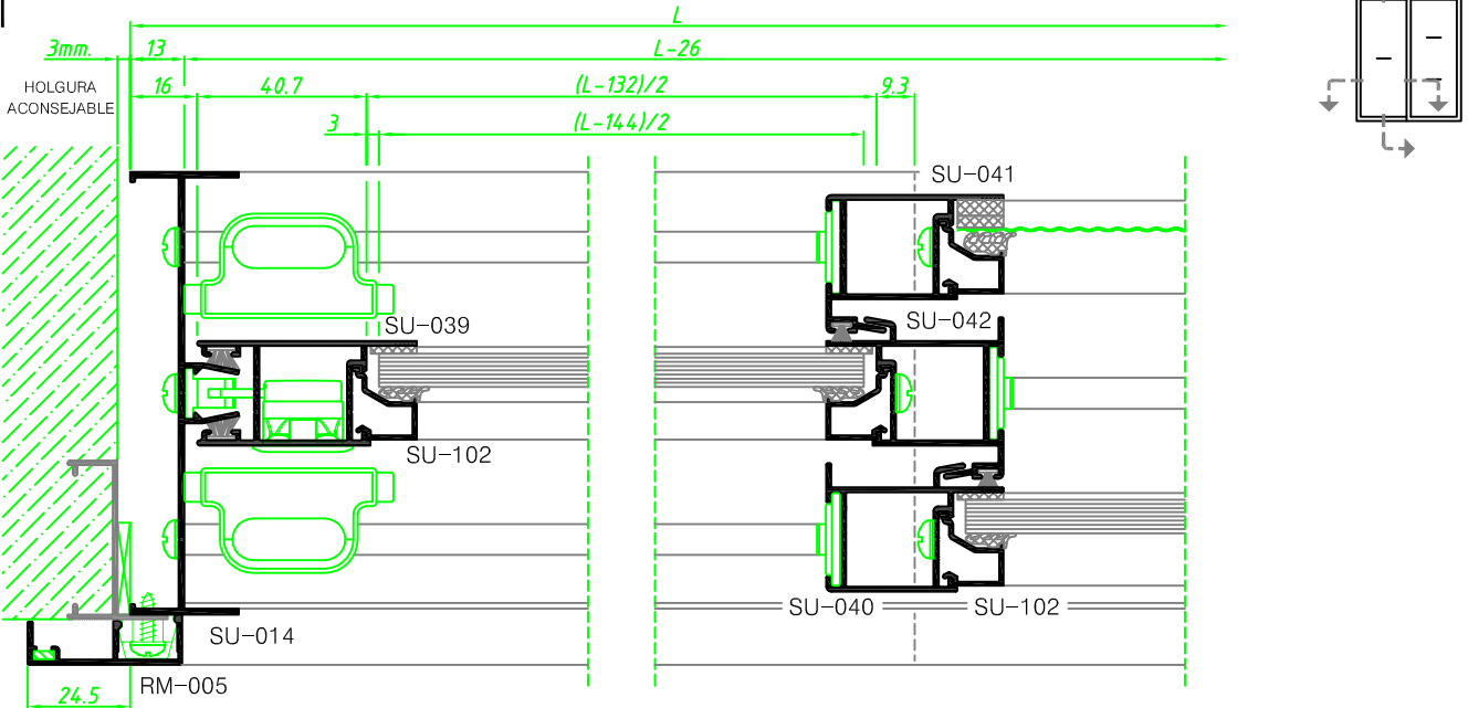
CORTE HORIZONTAL
