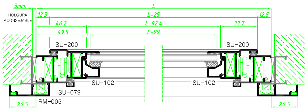
CORTE HORIZONTAL
