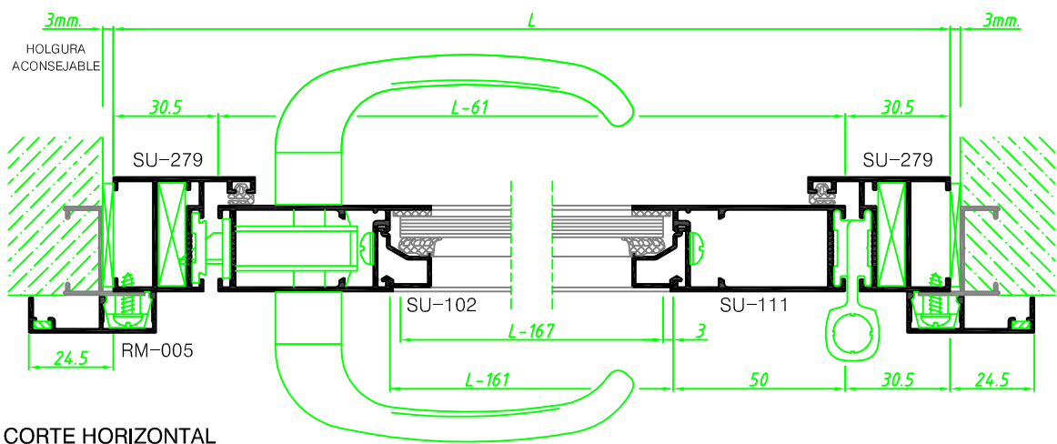
CORTE HORIZONTAL
