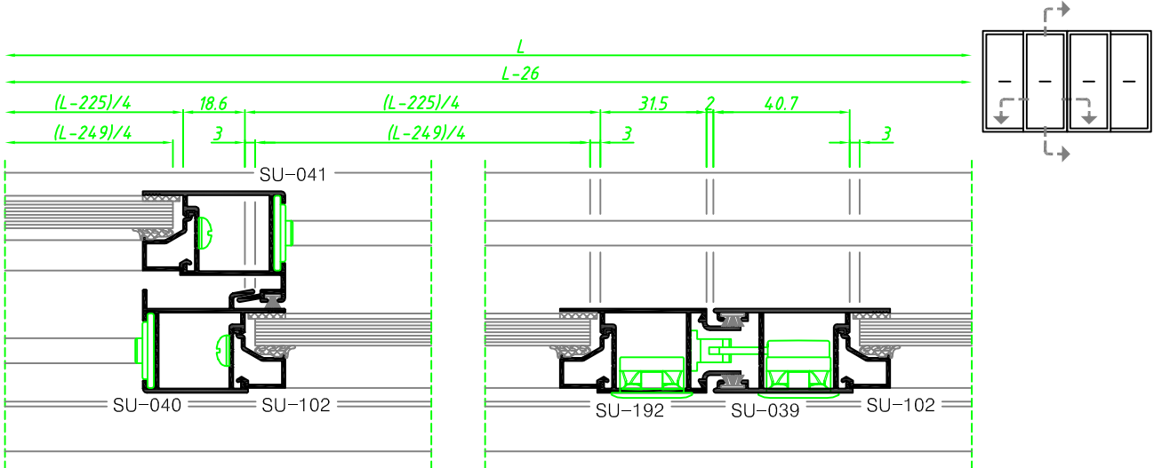
CORTE HORIZONTAL
