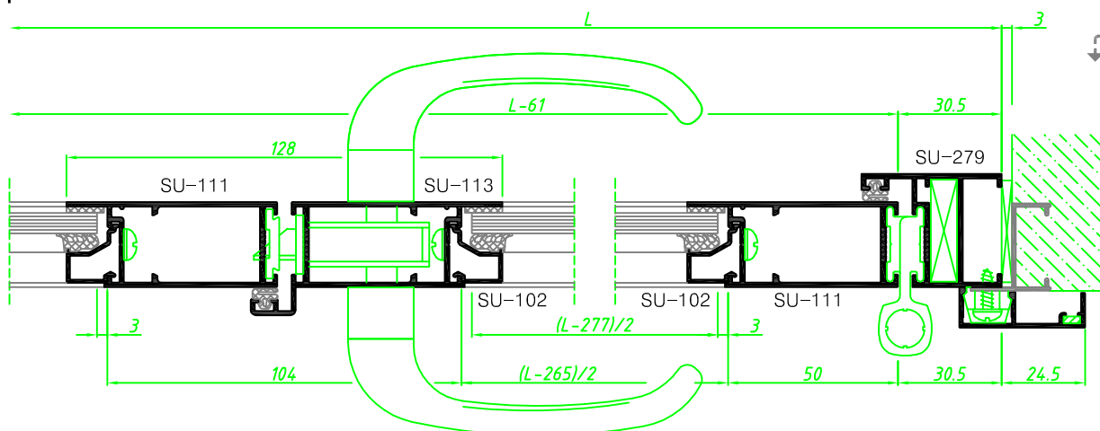
Encuentro inferior y central PUERTA BATIENTE de 1 y 2 HOJAS
