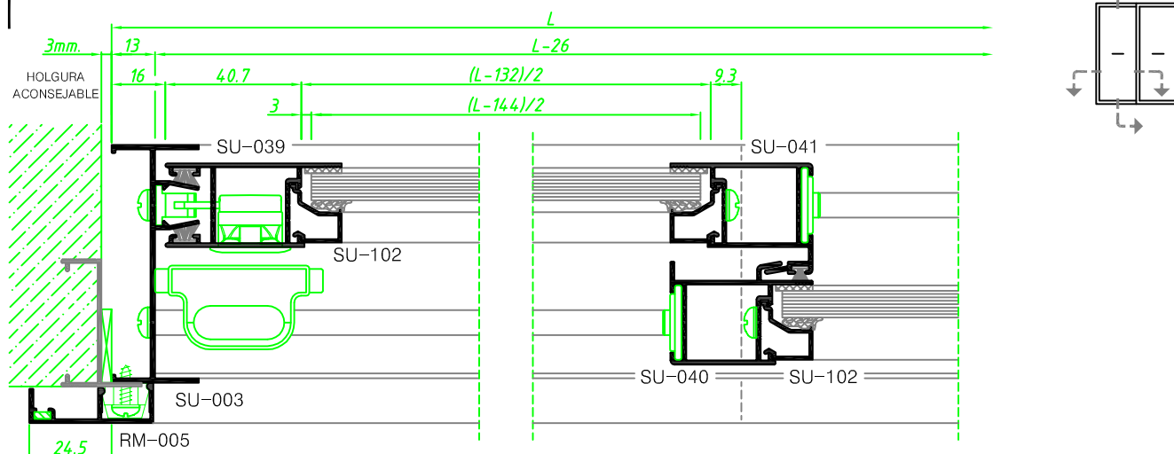
CORTE HORIZONTAL
